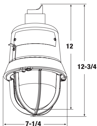
Pendant mount
